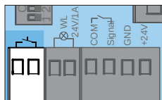
Fig. Conexión pulsador
